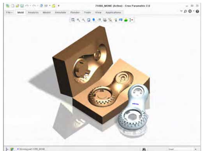
Fotorealistische PTC Creo Darstellung von Kernform und Kunststoffteilen
