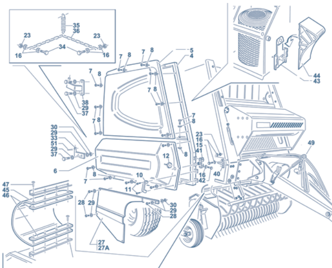
Abb. 21. Illustration mit indirekten Positionsnummern und Vergrößerungen mit freundlicher Genehmigung der Montanari Group, Correggio, ( www.montanarigroup.it )
