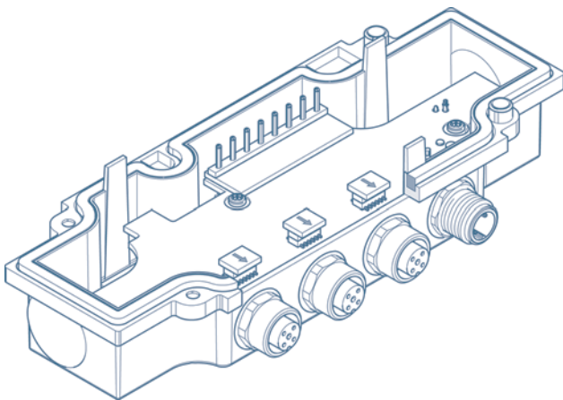
Abb. 15. Parallelperspektive in der praktischen Anwendung
